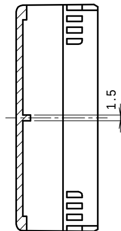
A-A断面図
